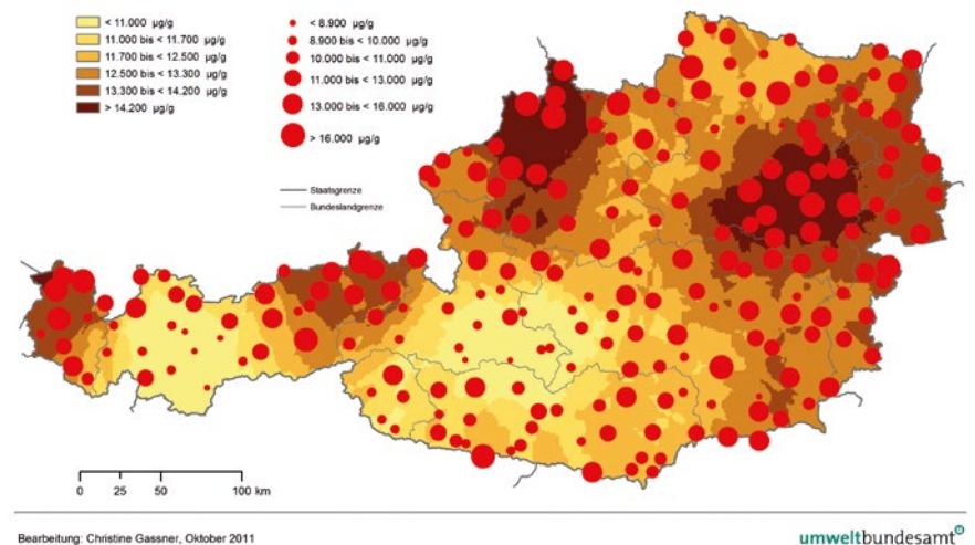
Abb. 47: Stickstoffgehalt von Moosen in Österreich (SCHRÖCK u. a. 2014).
